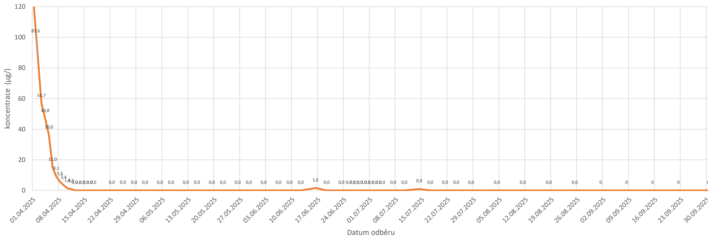
Vývoj koncentrace benzenu (µg/l) - povrchová voda profil 5
